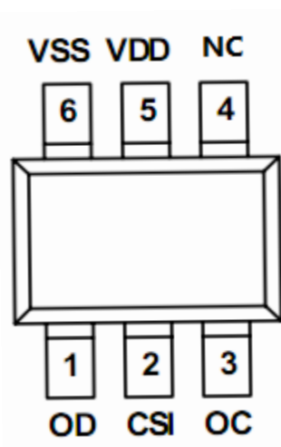
图1 FHDW01B 的 SOT23-6 封装及引脚排布
