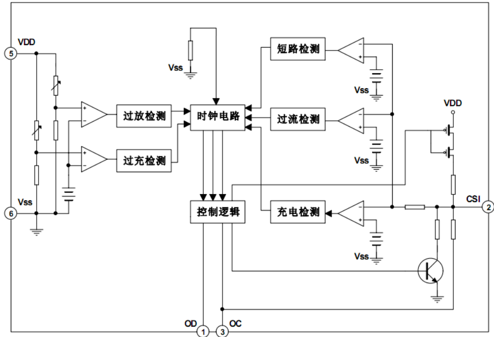
图2 功能框图
