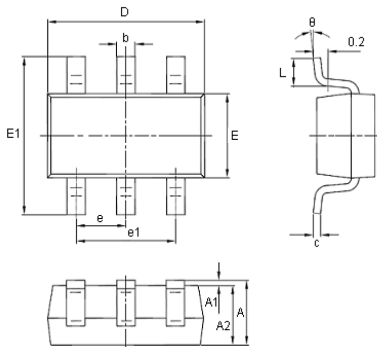
图-7 SOT23-6 封装外形尺寸图
