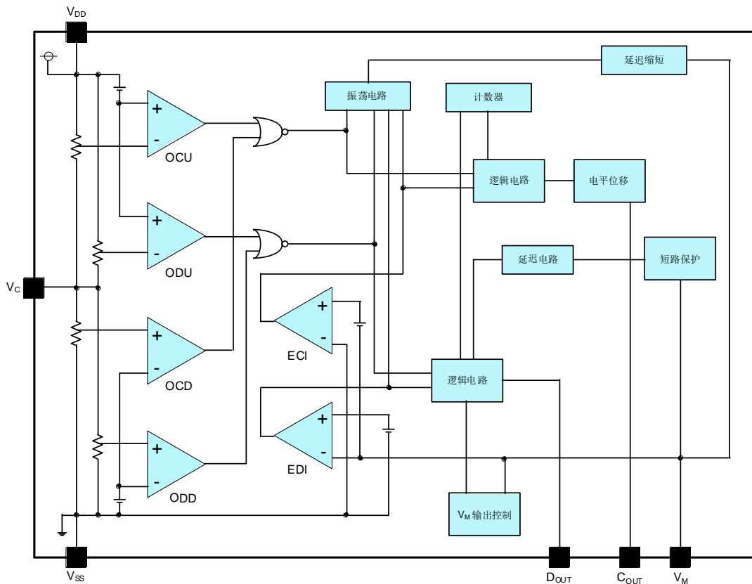
图-3 FH2120-OB 功能框图
