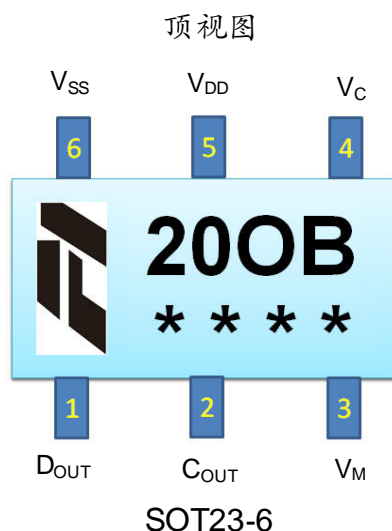
图-2 FH2120-OB 管脚排列 (*号丝印会变化)
