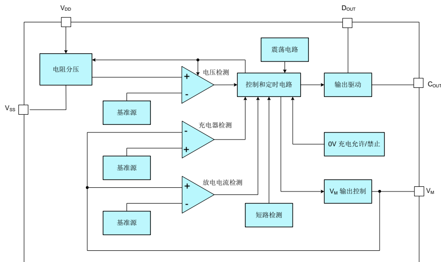
图-1 FH01 功能框图
